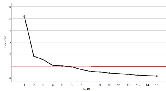
شکل ۲. نمودار سنگ‌ریزه
